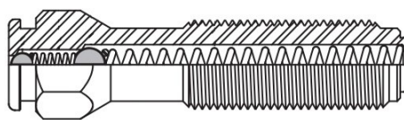
双球止回阀
