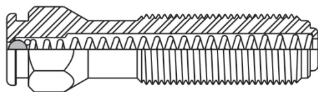
单球止回阀
