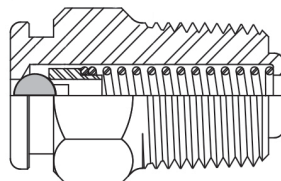
单球止回阀
