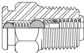
双球止回阀
